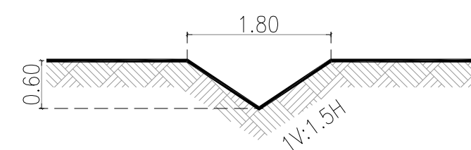
DETALLE SECCION CUNETA TIPO
