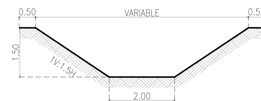
DETALLE SECCION CUNETA TIPO
