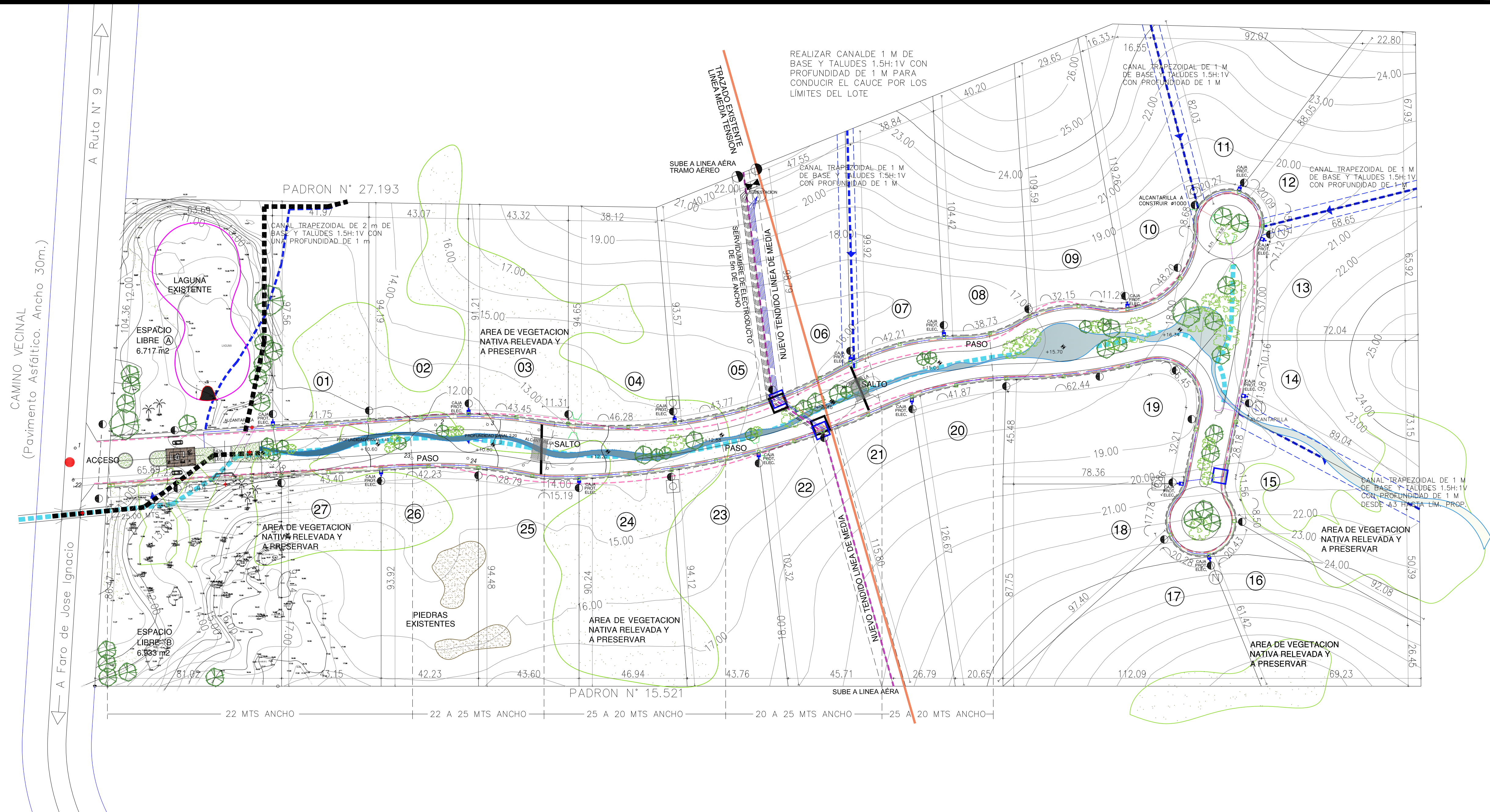
PLANO DE UBICACION
